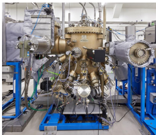
秘匿技術の中核となる量産型 MBE 装置
