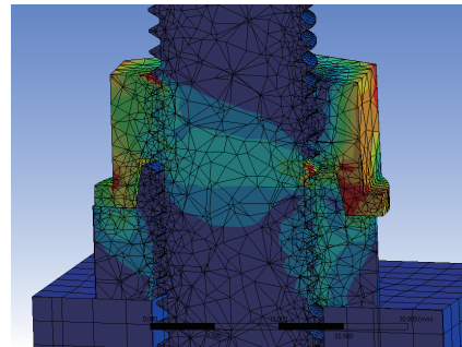
試作図面に基づいて理論的な評価を行ったFEM解析図
