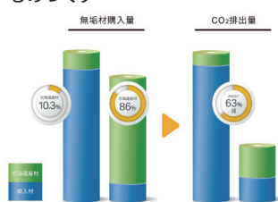
北海道産材購入量とCO 2 排出量の変化
