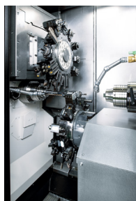
2タレット2スピンドル
