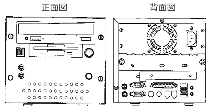
意匠登録第1164462号 「電子計算機」
