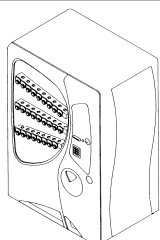
意匠登録第1116969号 商品自動販売機 意匠分類 J5-12B 意匠権者 三洋電機株式会社
