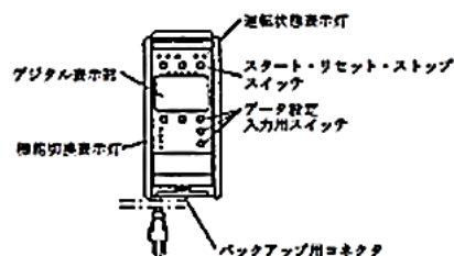
【操作部等を説明する参考正面図】
