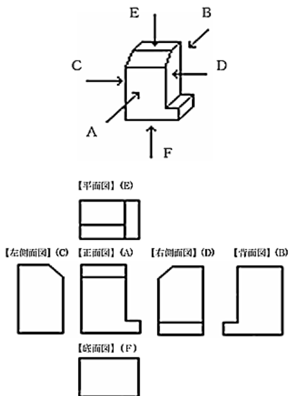
正投影図法の六面図の位置関係
