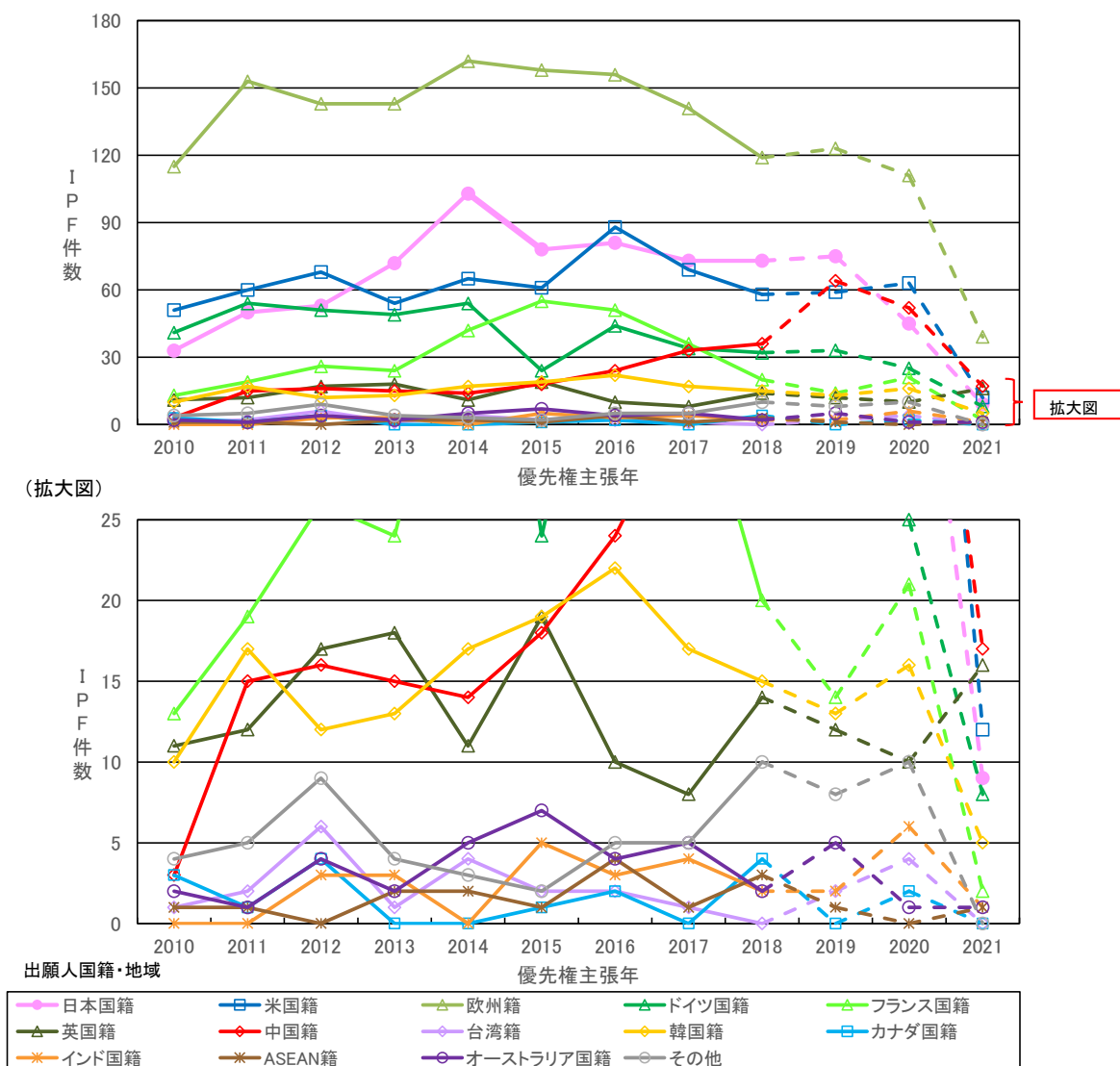
図 5-43 「gx03 : 熱エネルギー貯蔵」における出願人国籍・地域別 IPF 件数年次推移 (優先権主張年 2010 年～2021 年)
