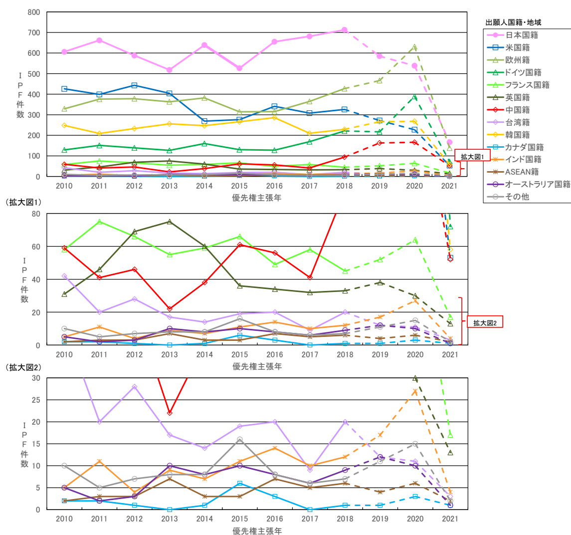
図 5-17 「gxA09：燃料電池」における出願人国籍・地域別 IPF 件数年次推移 (優先権主張年 2010 年～2021 年)
