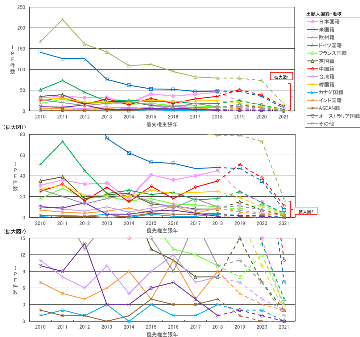
図 5-9 「gxA05：水力発電」における出願人国籍・地域別 IPF 件数年次推移 (優先権主張年 2010 年～2021 年)
