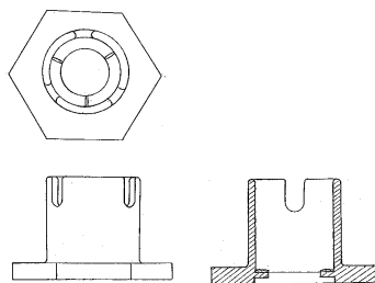
1170062 号 ボトル受け台
