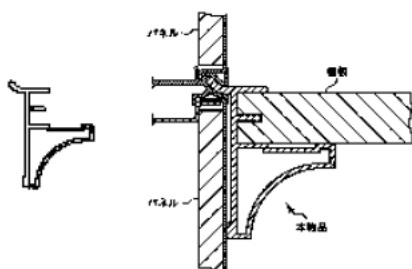
登録 1264387 「棚受金具」→D9-161
