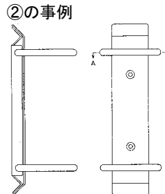
登録 930814 号 傘立て
