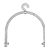
登録 1039030 植木鉢用吊り具
