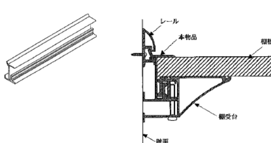
登録 1284995 「棚受金具用棚受台支持材」→D9-161
