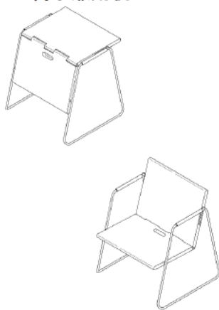
登録1194879号 椅子兼用机
