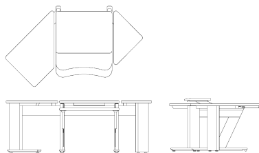
登録 01113399 電子機器載置用机
