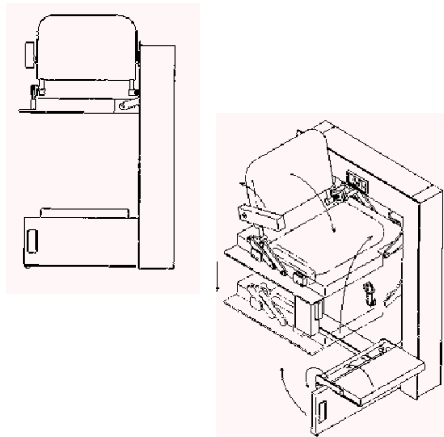
登録835784号 バスガイド用折畳みいす
