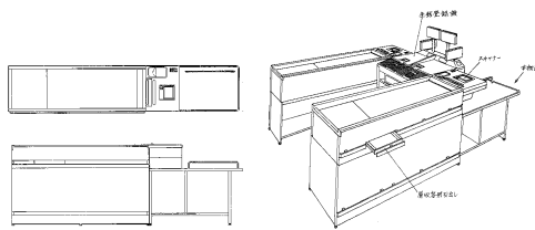
登録 00979882 チェックアウトカウンター
