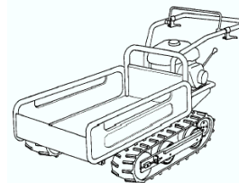
登録1033940号 運搬車 G2-200FA
