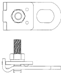
登録1135214号 電線分岐用引留金具
