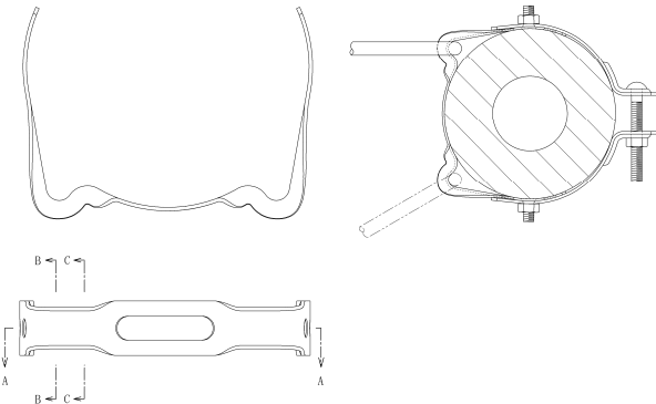
登録1341305号 支持線端部の電柱係止用バンド金具
