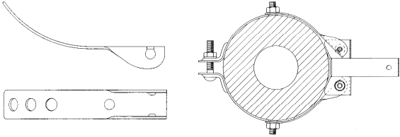
登録1183545号 電柱用バンド金具
