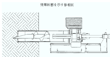
登録941958号 管削進機
