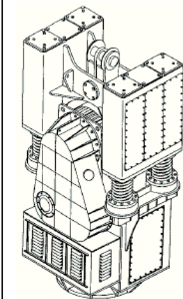
登録1170055号 くい打ち機用起振機
