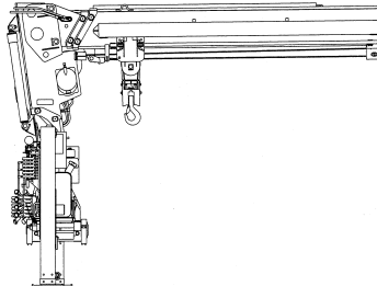
登録1446906号 車両搭載用クレーン G1-210
