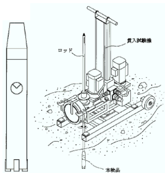
登録1087212号 土質サンプル採取用工具
