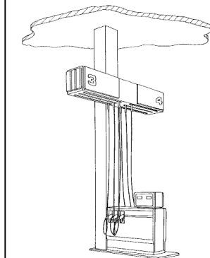
972065号 給油ホース吊下げケース
