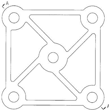
登録 886485 タイル連結用下板
