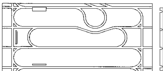
L6-104A 登録 1064038 号「床暖房用パイプ収納パネル」
