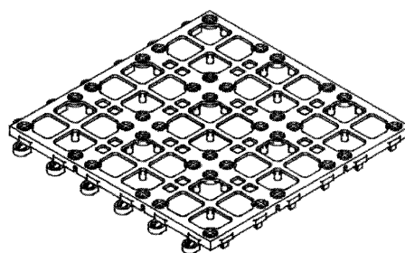
登録 1029119 タイル敷設用枠体
