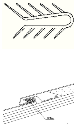
L6-1170 登録 1169505 号 「屋根用シーリング材」
