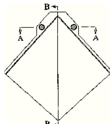
登録1070488棟隅がわら
