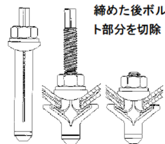
904432-1 コルゲート鋼板用締結金具
