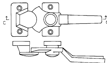
登録 0777032 薬品保管庫の扉用ハンドル
