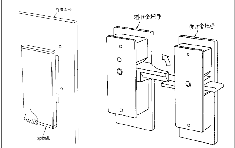
登録 0611152 門扉用把手
