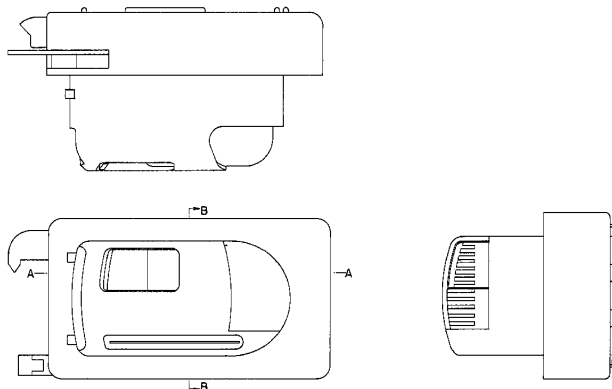
登録 0943087 家具用錠付き取手
