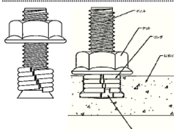
1143077 タイル固定用 拡張ボルトアンカー
