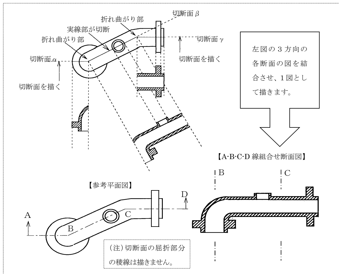
〔図 1.2-24〕【組合せ断面図】の考え方と記載例
