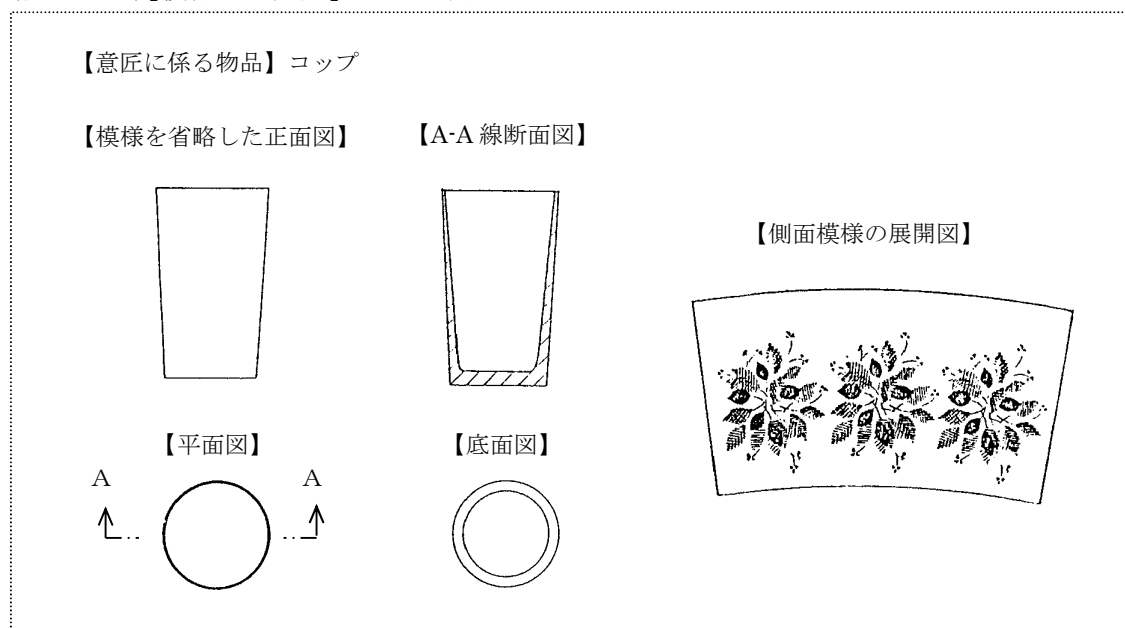
〔図 1.2-20〕【模様を展開図】を用いた例
