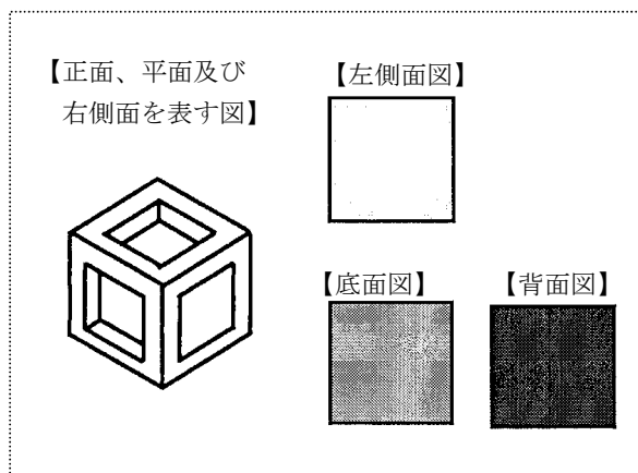
〔図 1.2-10〕正投影図法、等角投影図法併用例
