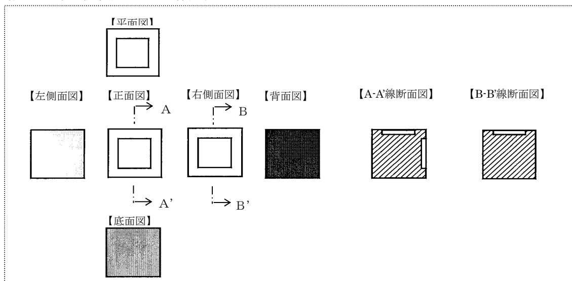
〔図 1.2-8〕正投影図法による作図例
