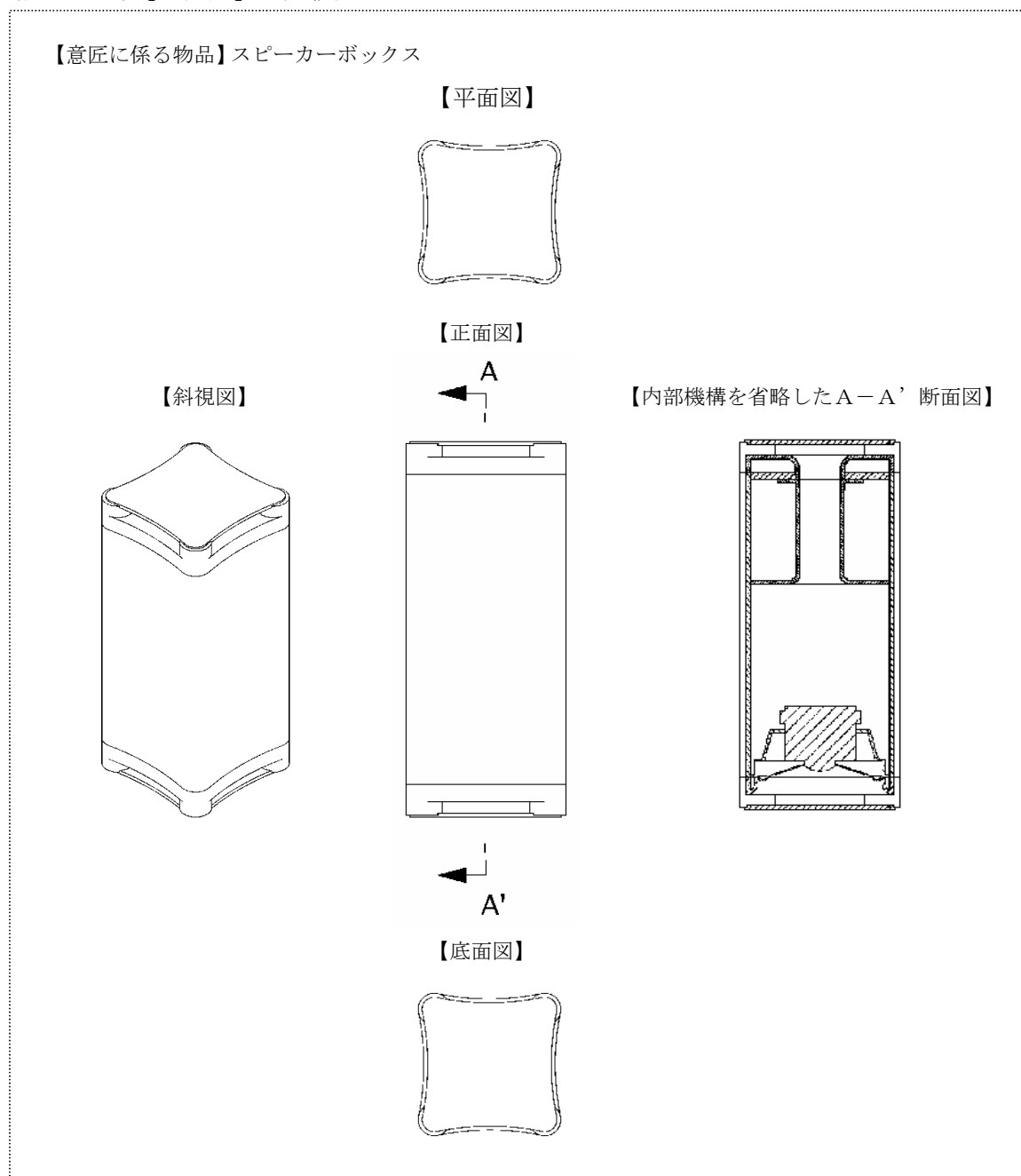
〔図 1.2-22〕【断面図】の記載例
