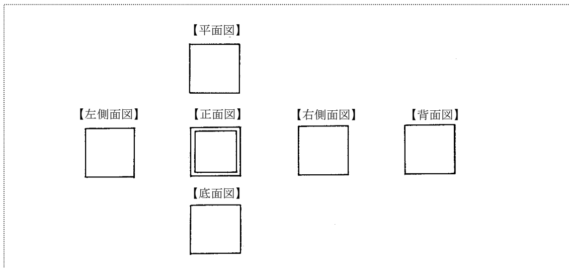
〔図 1.2-18〕一組の6面図のみの図面の例
