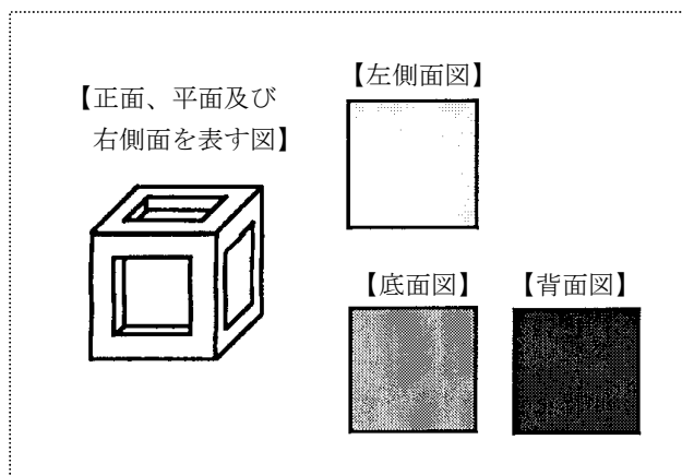
〔図 1.2-12〕正投影図法、キャビネット図併用例
