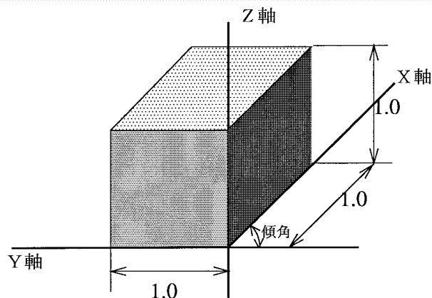
〔図 1.2-7〕カバリエ図による作図例
