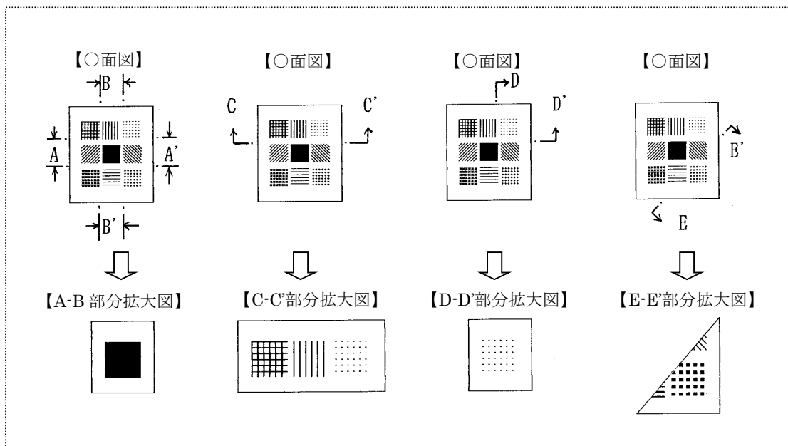
〔図 1.2-29〕部分の区切り方と指示線の記載例
