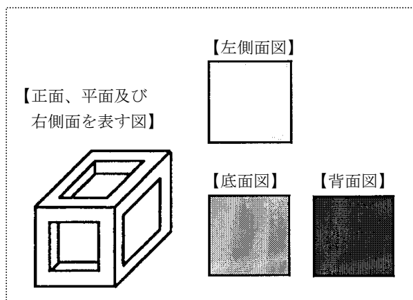
〔図 1.2-14〕正投影図法、カバリエ図併用例
