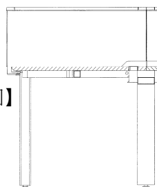
【B-B 拡大断面図】
