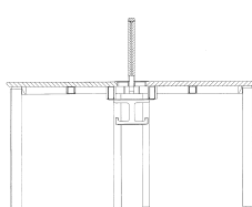
【B-B 拡大断面図】
