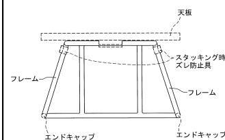
【各部の名称を示す参考図】
