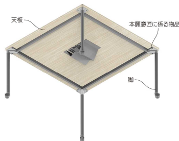
【使用状態を示す参考図】
