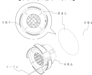
【使用状態参考図】
