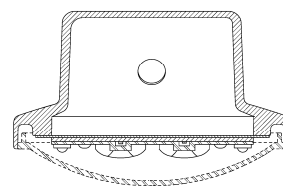
【内部機構を省略した B-B線拡大断面図】
