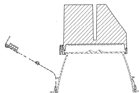
【内部機構を省略した A-A線端面図】
