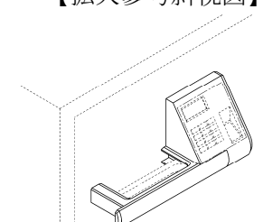
【拡大参考斜視図】
