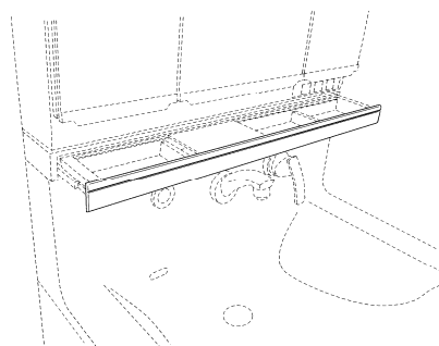
【使用状態を示す参考部分斜視図】
