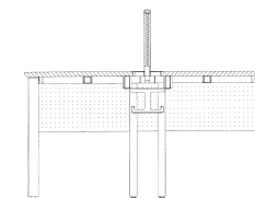
【B-B 拡大断面図】
