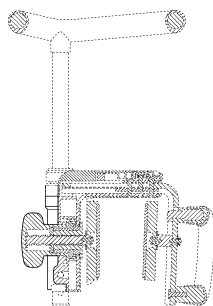
【B-B線断面図】
