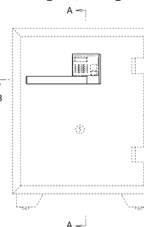
【正面図】
