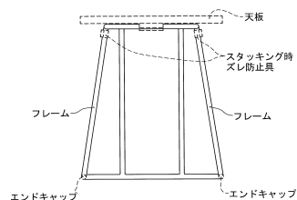
【各部の名称を示す参考図】
