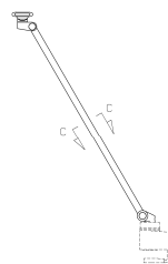
【内部機構を省略した B-B線端面拡大図】
