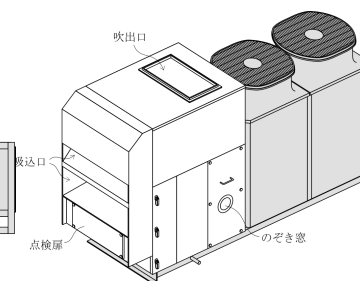
【各部の名称を示す 参考斜視図】
