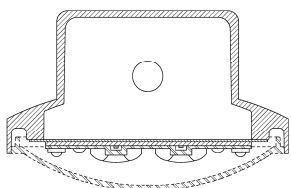
【内部機構を省略した B-B線拡大断面図】
