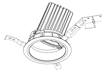
【斜視図 (1)】
