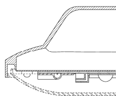
【C-C線、D-D線で 囲まれた部分の拡大図】
