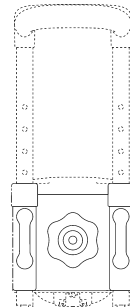
【左側面図】
