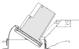
【内部機構を省略した A-A線断面図】
