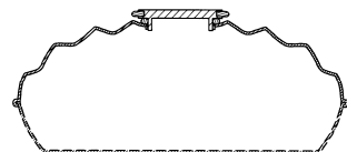
【A-A切断部端面図】
