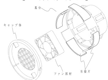
【参考分解斜視図】
