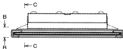
【内部機構を省略した A-A拡大断面図】
