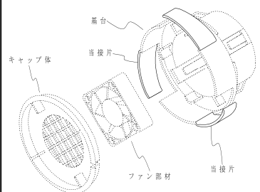
【参考分解斜視図】
