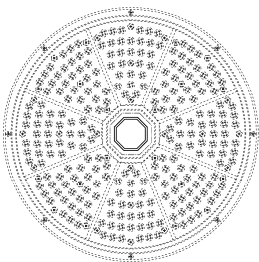
【底面図】
