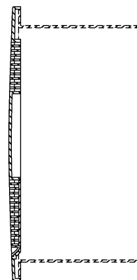
【内部機構を省略したA-A'断面図】
