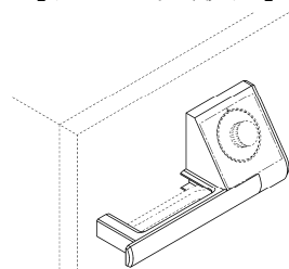
【拡大参考斜視図】
