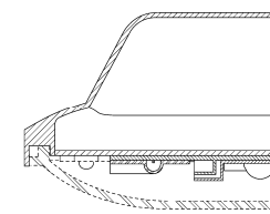
【C-C線、D-D線で 囲まれた部分の拡大図】
