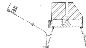
【内部機構を省略した A-A線端面図】
