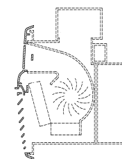
【内部機構を一部省略した A-A 切断部端面図】
