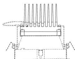
【内部機構を省略した A-A線端面図】
