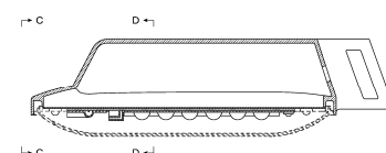
【内部機構を省略した A-A線断面図】
