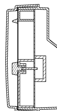
【内部機構を省略したA-A端面図】
