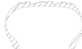
【C-C線端面図】
