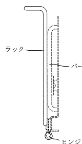
【各部名称を示す参考右側面図】
