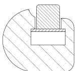
【内部構造を省略した B-B切断部端面拡大図】
