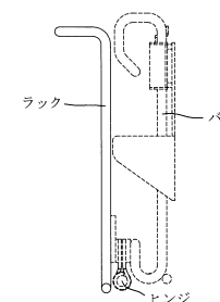
【各部名称を示す参考右側面図】
