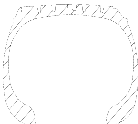
【B-B線端面図】
