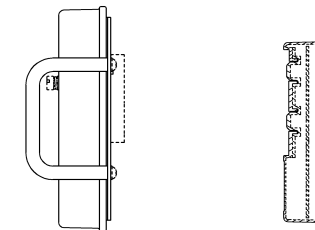
【内部機構を一部省略したA-A端面図】
