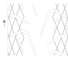
【正面図の部分拡大図】
