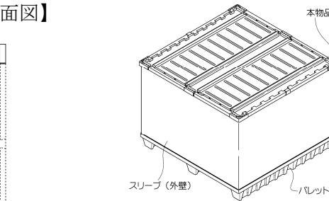
【正面、底面及び 右側面を表す図】
