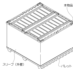
【正面、底面及び 右側面を表す図】
