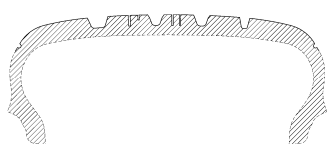
【C-C部A-A線 拡大端面図】
