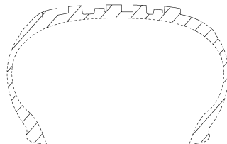
【C-C線端面図】
