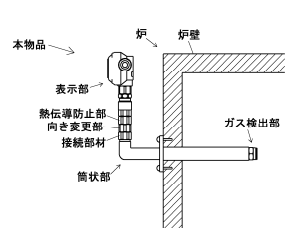
【使用状態を示す参考図 1】
