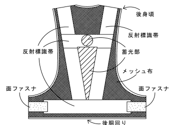
【構成を示す 参考背面図】
