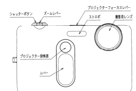
【各部の名称を 示す参考図】
