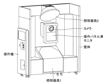
【名称を示す参考斜視図】
