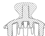
【正面図中央縦断面図】
