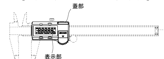
【全表示素子を表した参考正面図】
