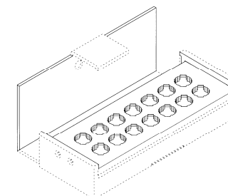
【蓋を開いた状態の斜視図】
