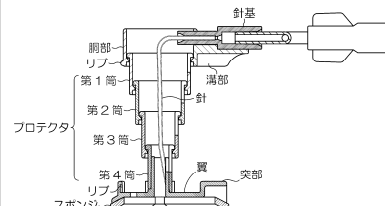
【各部の名称を示す参考図】
