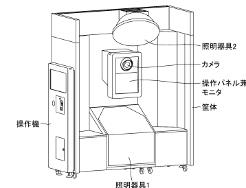
【名称を示す参考斜視図】
