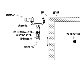
【使用状態を示す参考図 2】
