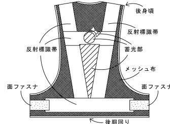
【構成を示す 参考背面図】
