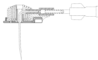
【A-A線断面図】
