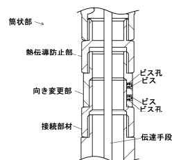
【拡大参考断面図】
