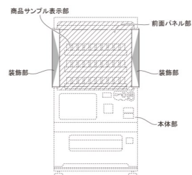
【透明部分及び各部名称を示す参考正面図】
