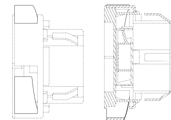
【右側面図】
