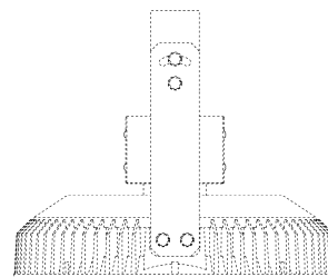
【左側面図】
