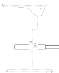
【右側面図】
