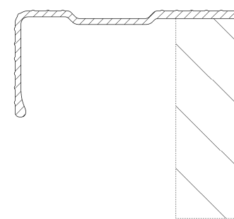
【B-B部分の拡大図】
