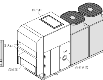
【各部の名称を示す 参考斜視図】
