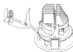
【斜視図】
