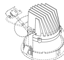
【斜視図】
