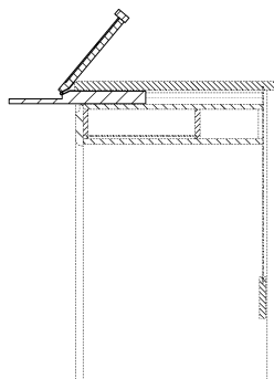
【A-A断面図】
