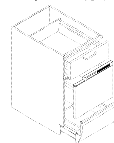
【扉を開けた状態の斜視図】
