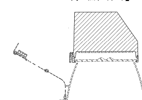
【内部機構を省略した A-A線端面図】
