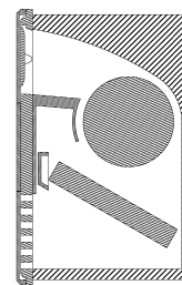
【内部機構を省略した参考 A-A 断面図】
