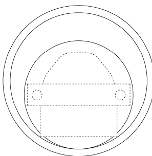
【内部機構を省略したB-B線断面図】
