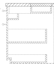
【右側面図】
