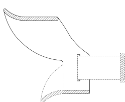
【A-A断面図】
