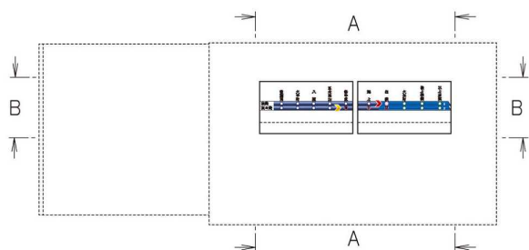
【正面図】
