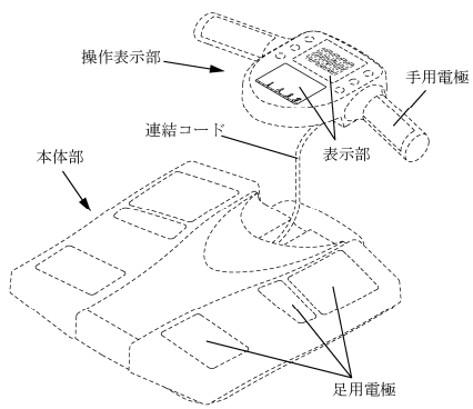
【各部名称を示す参考斜視図】
