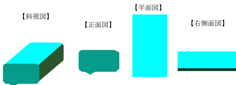
意匠に係る物品「消しゴム」
