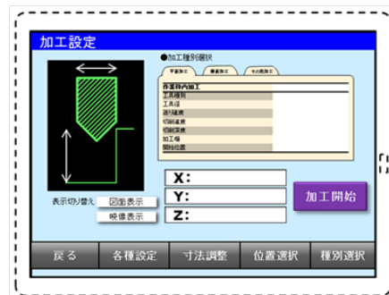
「マシニングセンタ制御機能付き 電子計算機」 (切削加工内容の設定を行うための画像)
