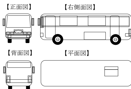
意匠に係る物品「バス」 【意匠の説明】 左側面図は右側面図と対称につき省略する。
