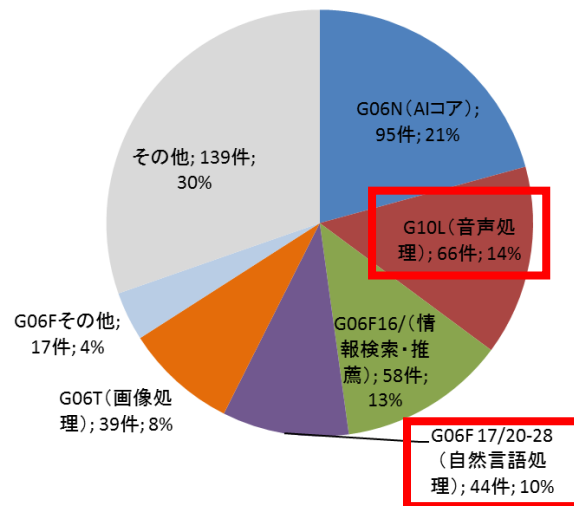
図 11-2 RNN 又は LSTM に言及する AI 関連発明の主分類構成 (2013-17 年出願)
