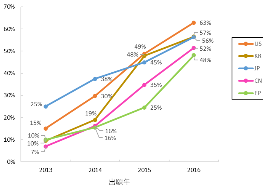
図 16 G06N3/02-3/10 が付与された各国出願のうち、 出願書類中に深層学習関連キーワードを含むものの割合の推移
