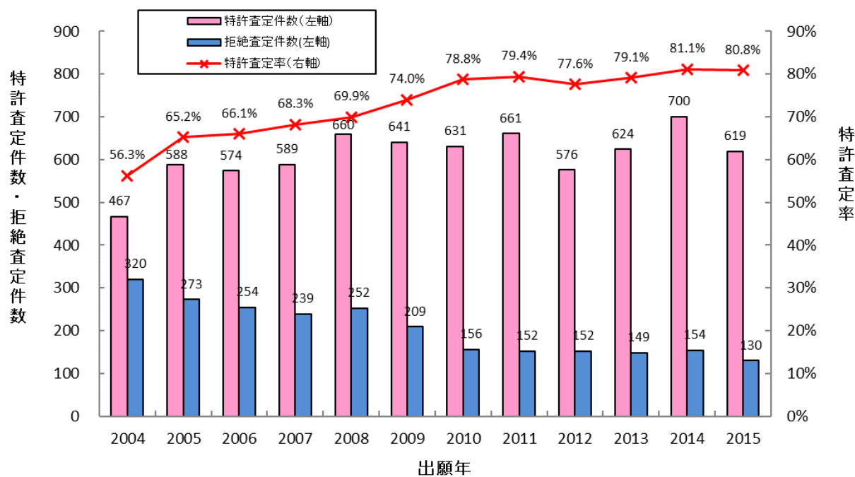
図 6 AI 関連発明の特許査定率の推移
